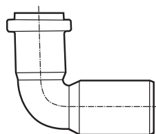
HTRB 50/40 Curva ridotta con guarnizione tipo 50/A o 50/B
