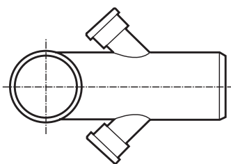
HTSB-Do-40 HTSB-Do-50 Curva WC doppia con guarnizione con due attacchi Ø 40 o Ø 50
