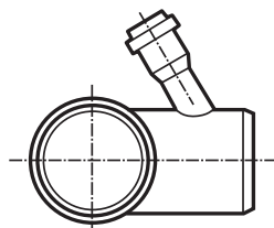
HTB-S-40 HTB-S-50 Curva grigia con attacco sinistro Ø 40 o Ø 50
