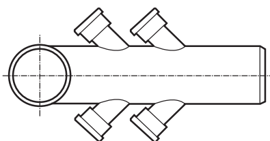
HTSB-4A-40 HTSB-4A-50 Curva WC con guarnizione con quattro attacchi Ø 40 o Ø 50
