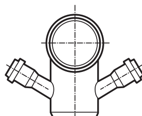
HTB-Do-40 HTB-Do-50 Curva grigia con due attacchi Ø 40 o Ø 50
